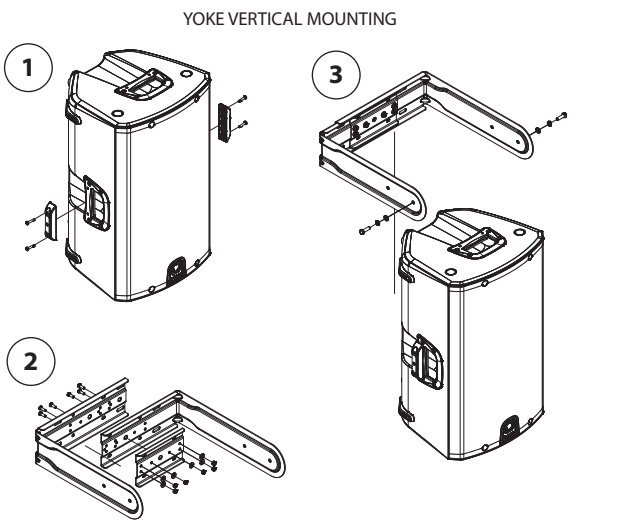
Krok 2: Montaż stalowego wspornika jarzma: iQ8 i iQ10
