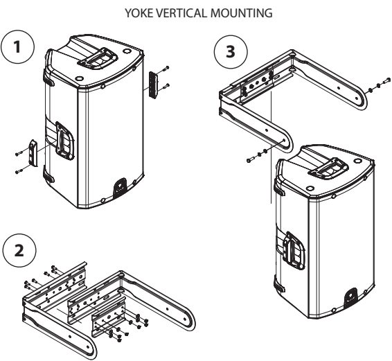
Etapa 2: Monte o suporte do garfo de aço: iQ8 e iQ10
