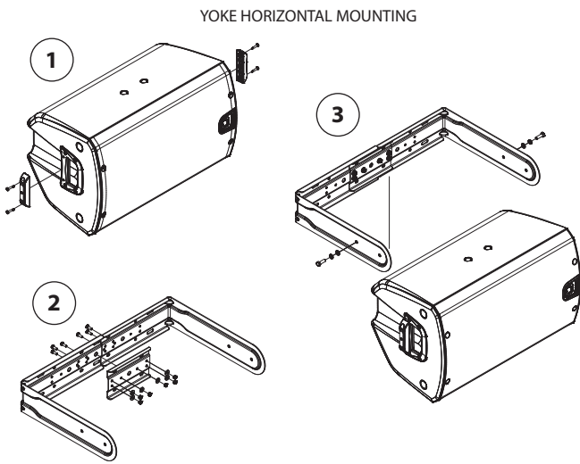
Steg 1: Fäst ok -distanser
