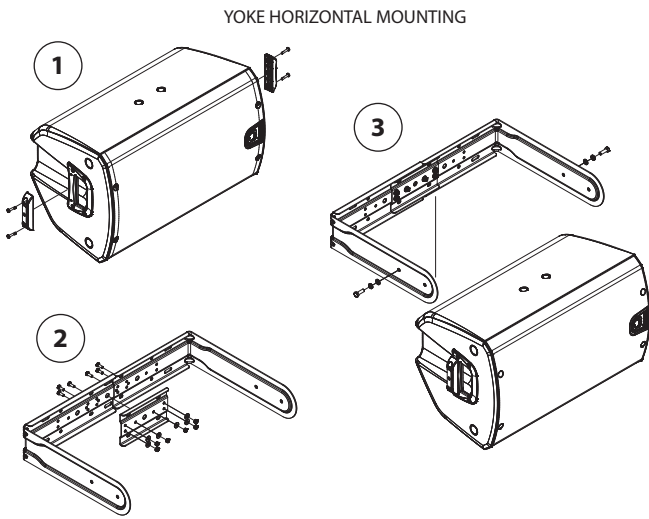
Passaggio 1: distanziatori del giogo sicuro
