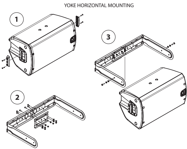
Etapa 1: prenda os espaçadores do garfo
