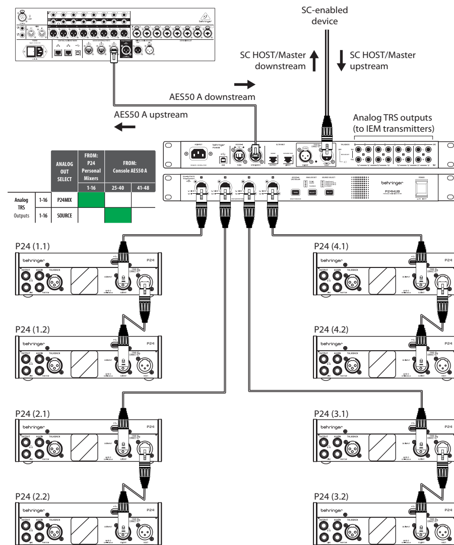
图 2: AES50 (24 通道) 作为源
