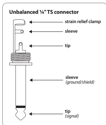
Fig. 2.2: Connettore jack TS da 1/4"
