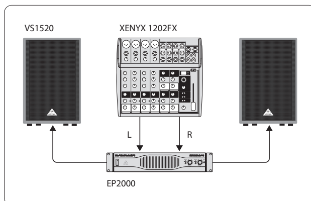
Fig. 5.1: Sistema stereo Full-range
